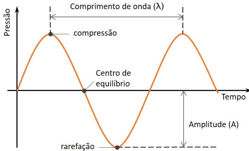
Figura 2.1: Amplitude da onda sonora.
