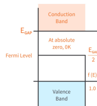
Gambar IV.1: Tingkatan Fermi pada Bahan Semikonduktor
