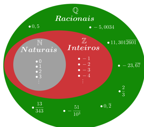
Figura 2 – Conjuntos
