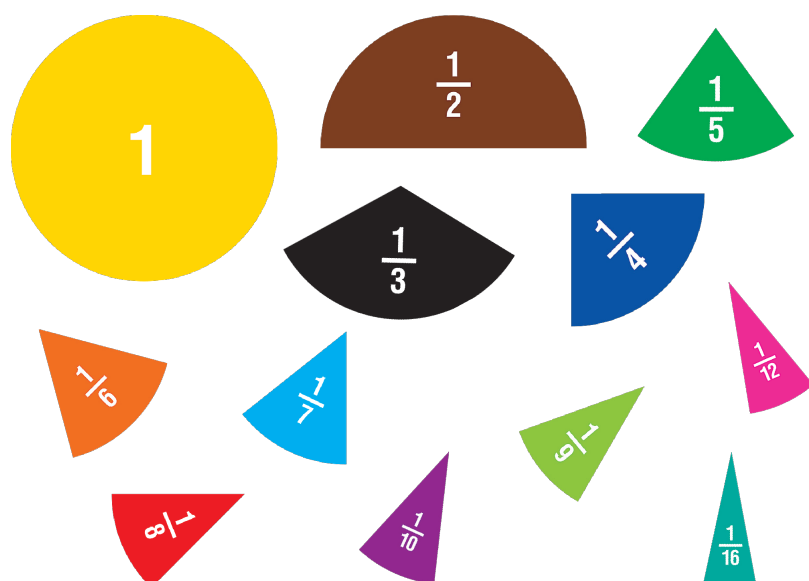
Figura 3 – Frações
