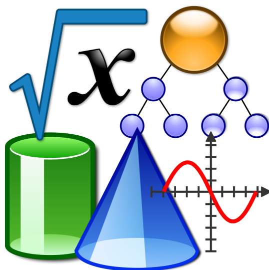
Figura 1 – Referências Matemáticas
